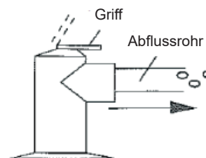
Druck- und Temperaturentlastungsventil
