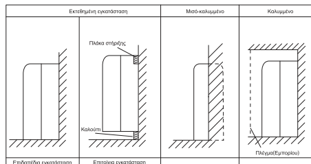
Ασφαλή τοποθέτηση για την εγκατάσταση της εσωτερικής μονάδας
