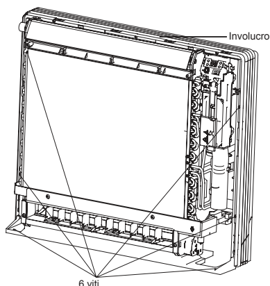
Installazione a pavimento
