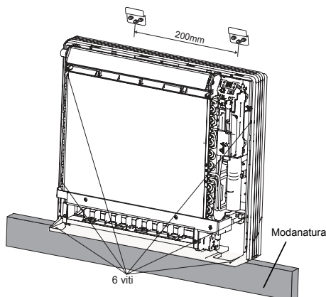
Installazione a muro
